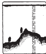
Interferenza elettrica
